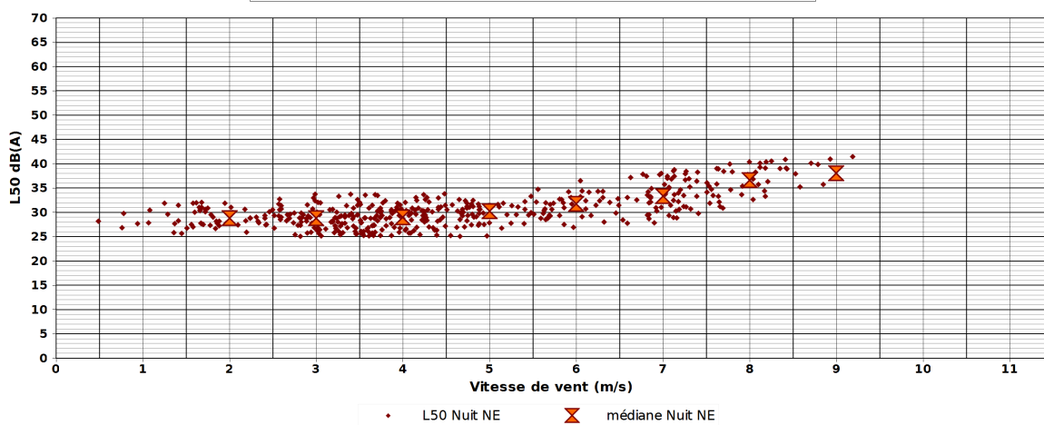
Point 11 : Les Champs - Secteur NE - Période Nuit - dB(A)
