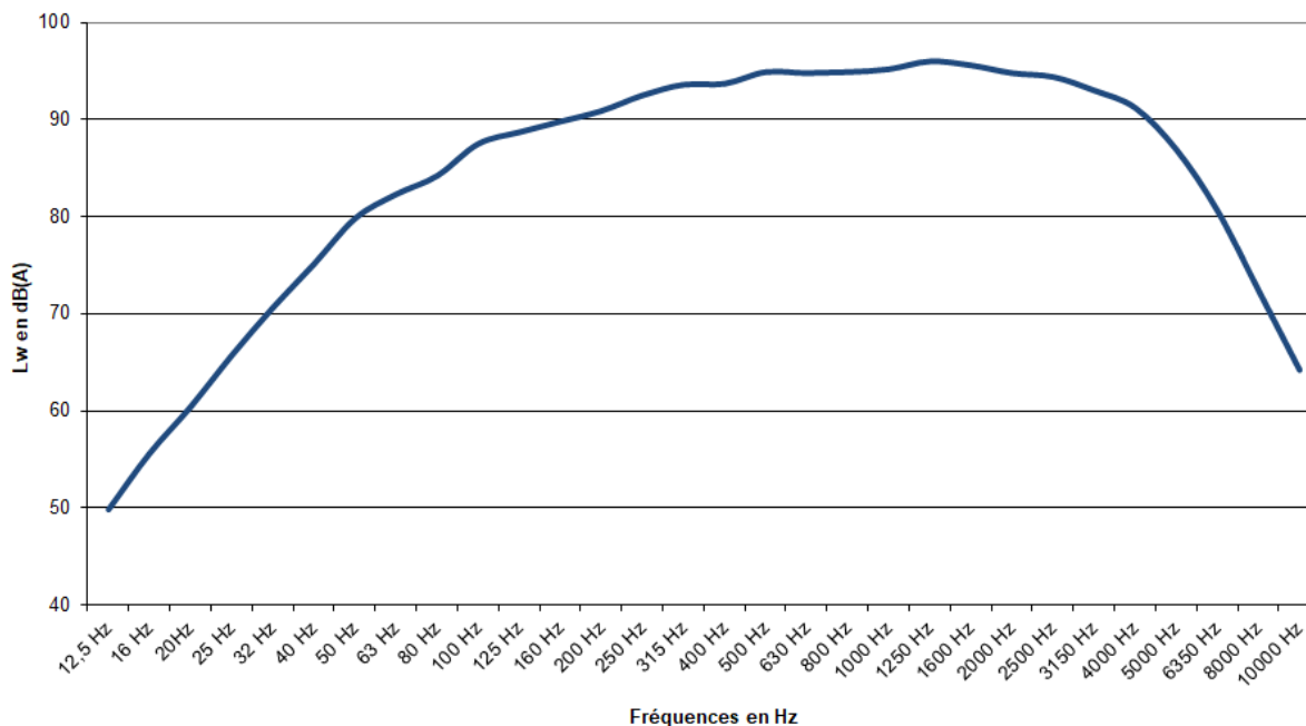
Spectre d'émission Vestas V110 2,2 MW STE mât de 95 m - 8 m/s à 10m
