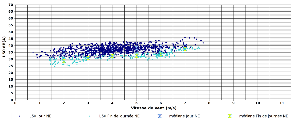
Point 11 : Les Champs - Secteur NE - Période Jour - dB(A)
