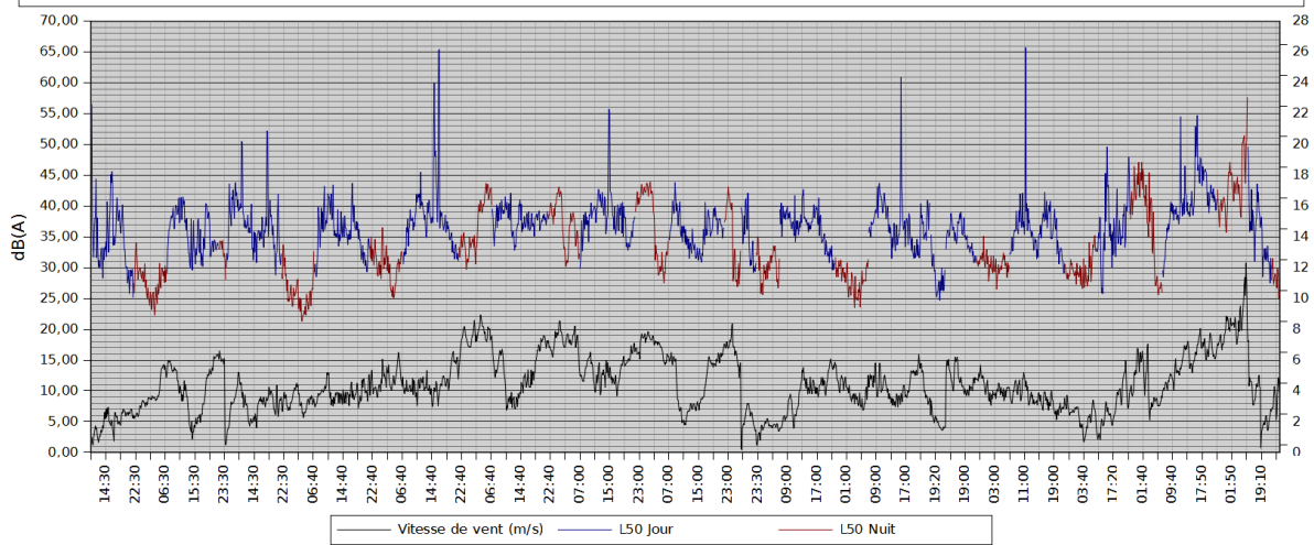
Evolutions temporelles ( dB(A) / Vent ) - Point 11 : Les Champs - Secteur NE - Période Jour/Nuit
